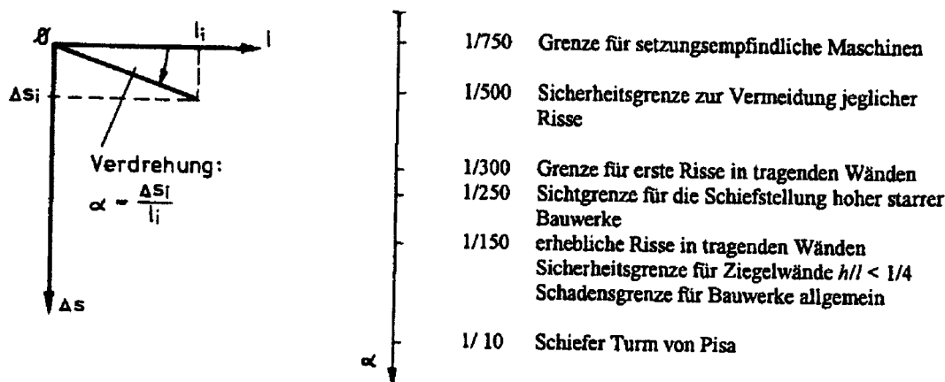
Abbildung 5-8: Grenzwerte für Verformungen bei Ausbildung einer Setzungsmulde
