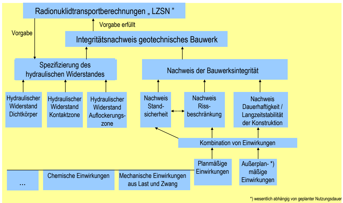
Abbildung 5-3: Zusammenhang zwischen Langzeitsicherheitsanalyse und dem ingenieurtechnischen Nachweis geotechnischer Barrieren
