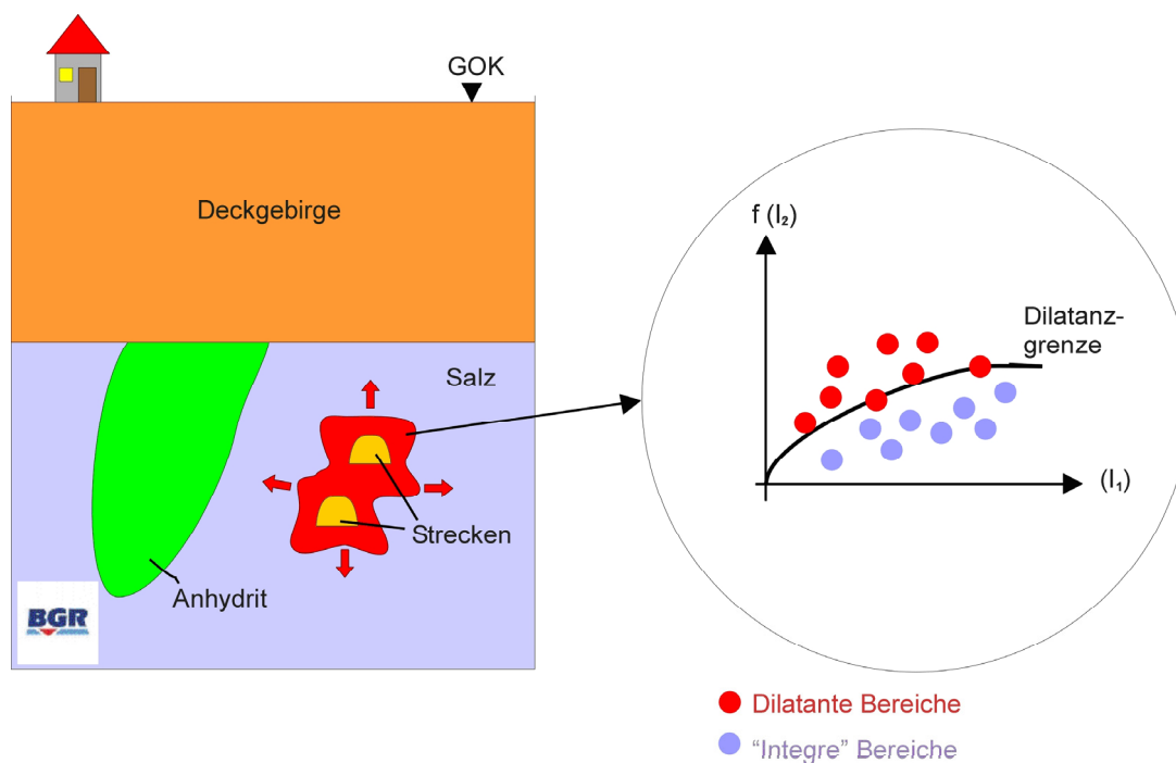
Abbildung 5-1: Visualisierung des Dilatanzkriteriums, dilatante Bereiche in der Barriere infolge bergmännischer Eingriffe
