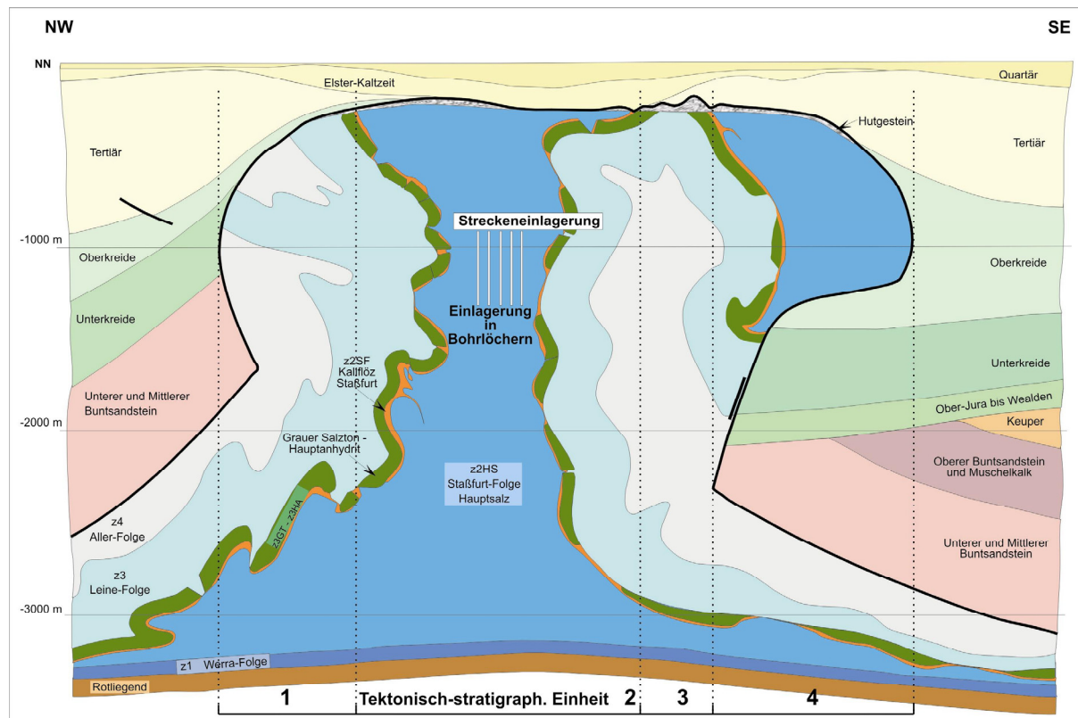
Abbildung 2-1: Vereinfachter, schematischer Schnitt durch den Salzstock des Referenzstandortes [Bornemann 2004].
