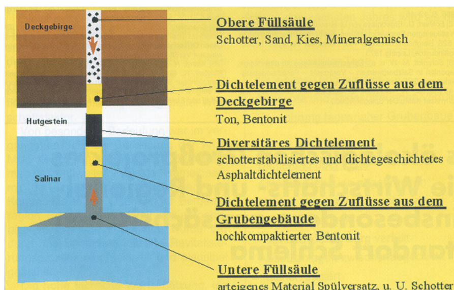
Abbildung 5-4: Vorschlag für ein Schachtverschlusskonzept für Endlager im Salinar
