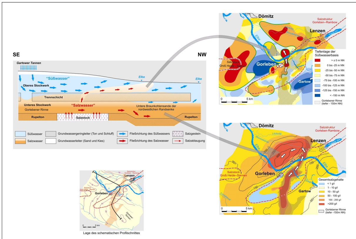
Abbildung 2-2: Schema des Salzwassertransports aus der Gorlebener Rinne [Klinge 2004]
