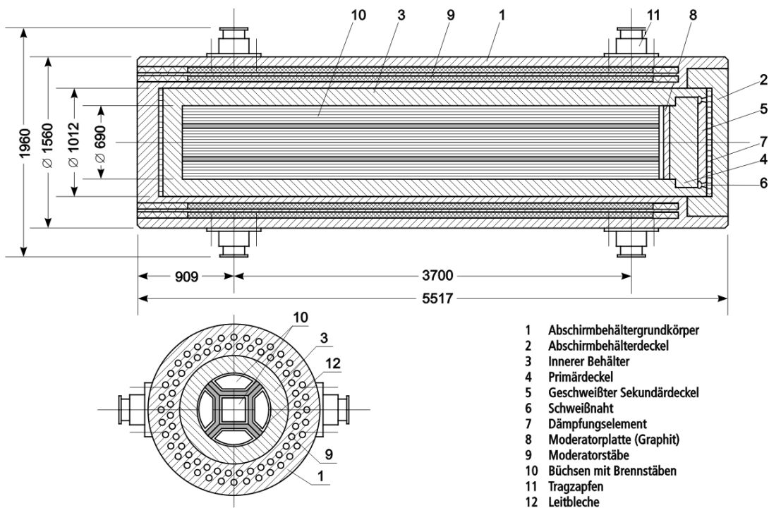
Abbildung 3-2: POLLUX-Behälter
