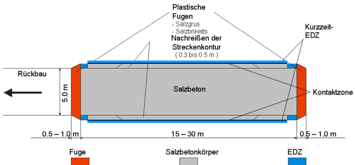
Abbildung 5-5: Entwurf Streckenverschluss ERAM
