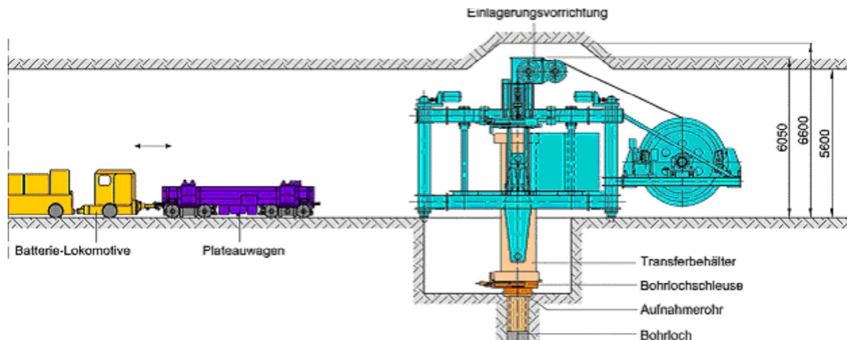
Abbildung 3-7: Komponenten des Einlagerungssystems zur Erprobung der Transport- und Einlagerungstechnik für BSK 3
