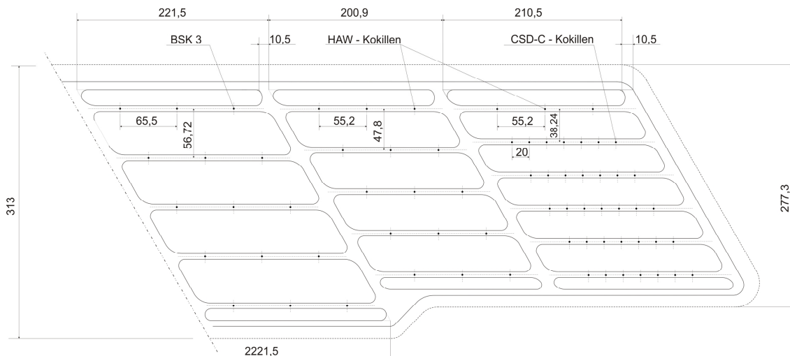
Abbildung 3-5: Grubengebäude für reine Bohrlochlagerung
