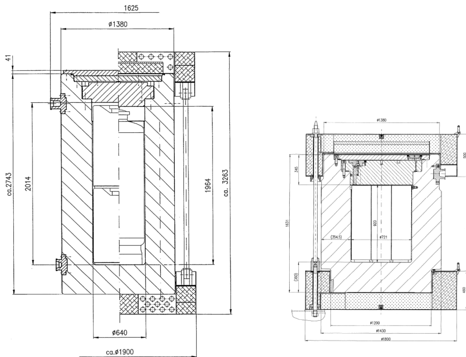
Abbildung 3-3: CASTOR AVR/THTR, links, (entspricht im wesentlichen auch CASTOR KNK) und CASTOR MTR 2, rechts
