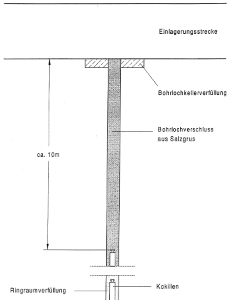
Abbildung 5-6: Bohrlochverschluss aus Salzgrus
