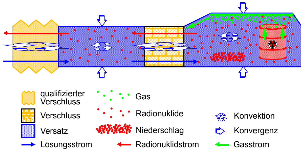
Abbildung 5-7: Teilmodell eines Grubengebäudes in LOPOS
