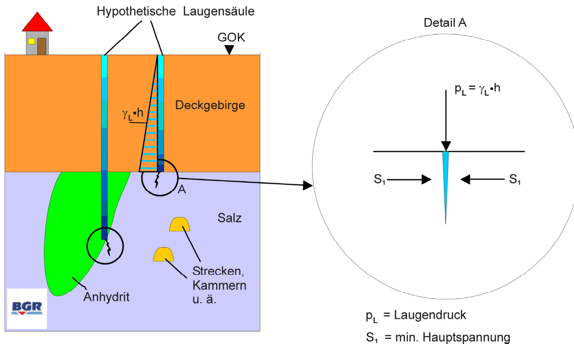
Abbildung 5-2: Visualisierung des Laugendruckkriteriums, Einwirkung von Laugendruck auf die geologische Barriere
