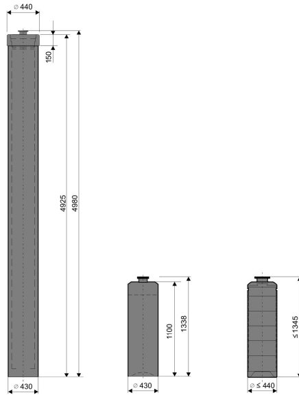
Abbildung 3-1: Brennstabkokille (BSK), links, HAW-Kokille, Mitte, (CSD-V, entspricht auch CSD-B) und CSD-C, rechts
